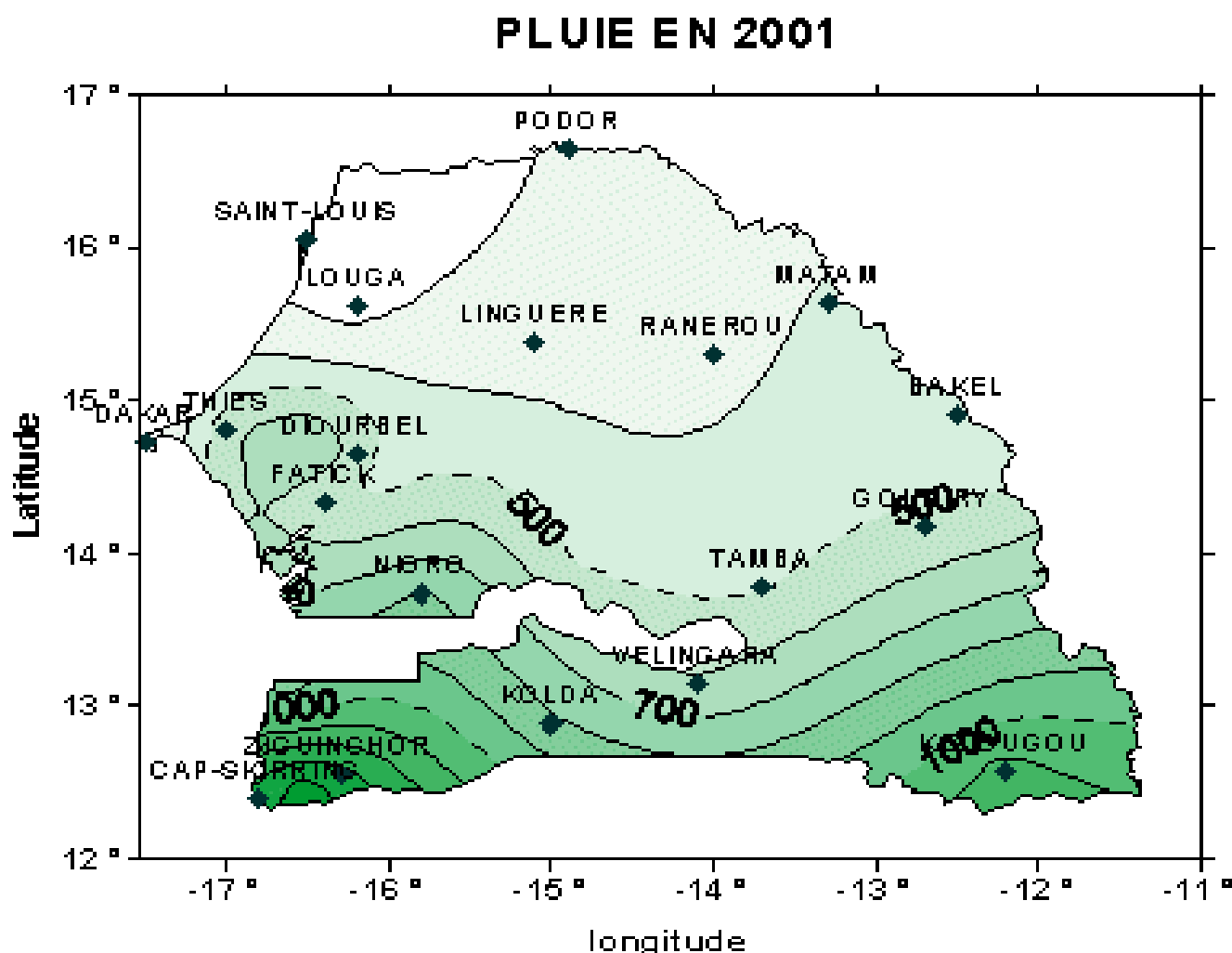
Figure 2- 4 : Cartes de la pluviométrie au Sénégal en 2001
